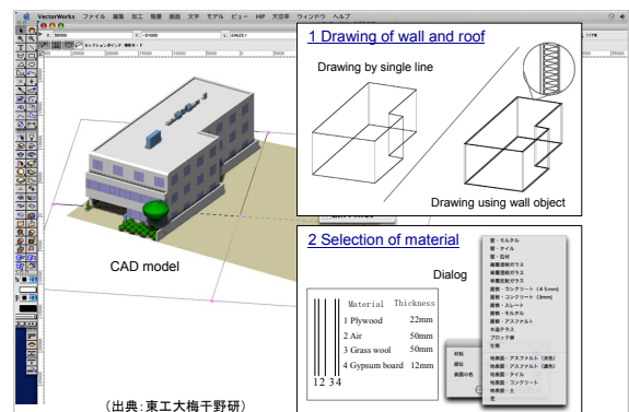
図7 ツール上での実際の作業画面の例(建物壁体における断面構成・物性の入力)
